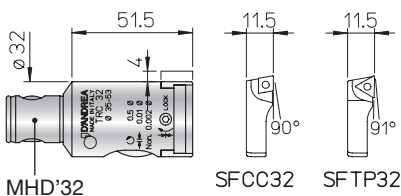
MHD'32
