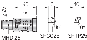
MHD'25
