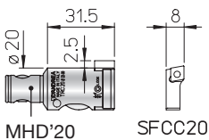
MHD'20
