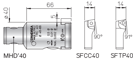
MHD'40
